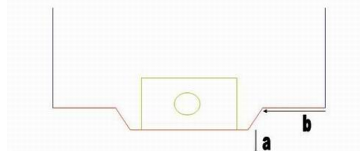
a: distancia mínima chasis a pista b: laterales del chasis a enrasar con la carrocería (mín 10mm.)
